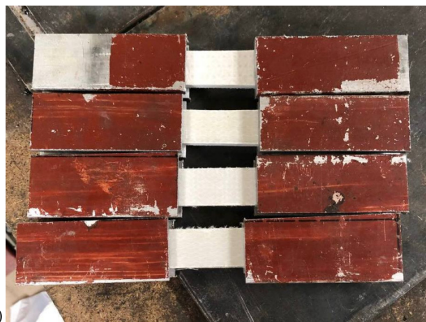
Рисунок 5 - Образцы с приклеенными алюминиевыми накладками
