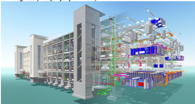
Рис. 1. Визуализация объекта строительства ( https://investcomtech.ru/raznoe-2/chto-takoe-bim-proektirovanie-bim-tehnologii-eto-prostym-yazykom.html )
