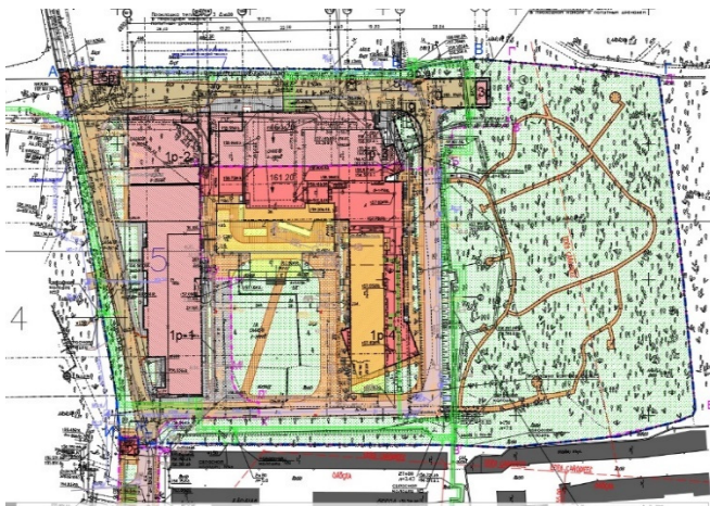
Рис. 7. Генеральный план Центрального госпиталя ФТС после реконструкции.
