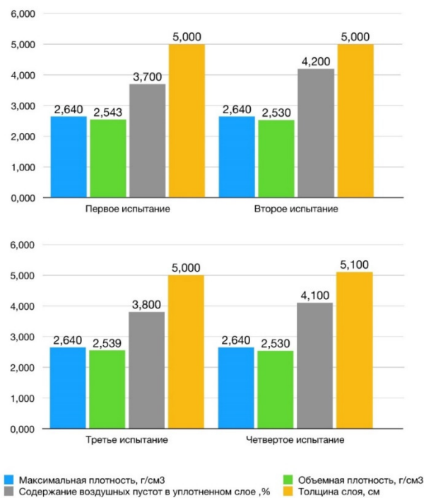
Рисунок 4- Результаты испытаний кернов готового покрытия из асфальтобетонной смеси SP-11Т
