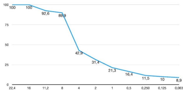
Рисунок 5 – График зернового состава минеральной части
