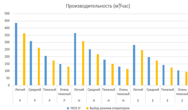
Рис. 2. Зависимость производительности от режимов работы
