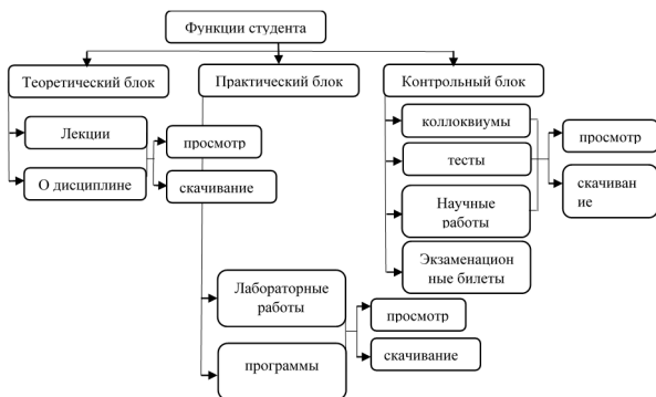
Рисунок 4 - Основное дерево функций системы обучающей микросети «Система-студент»
