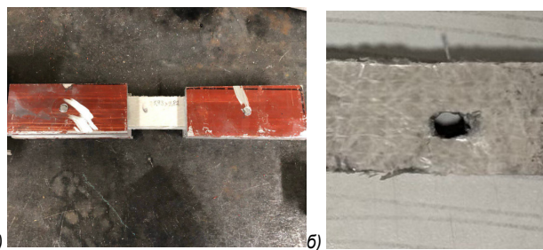
Рисунок 4 - а) образец с использованием алюминиевых накладок с предварительным сверлением в них и в образце отверстий под нагели б) скалывание в гнезде пластины
